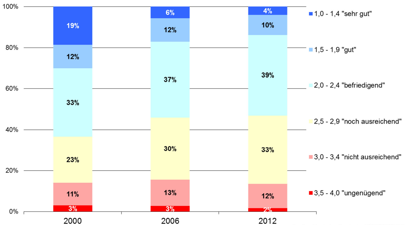
Zustandsbewertung nach Anteilen an Brückenflächen
